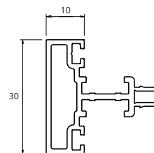
Tussenprofiel
