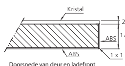
Doorsnede van deur en ladefront
