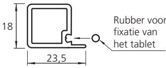
Profiel B voor drager
