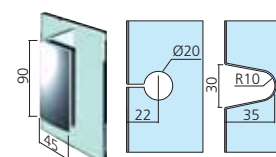
Scharnier glas/glas
