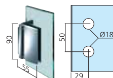
Scharnier muur/glas binnenkant
