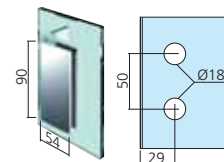
Scharnier muur/glas
