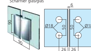
Scharnier glas/glas
