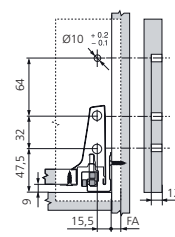
Inbouwmaten front (schroefmontage)
