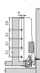
Inbouwmaten rugwand
