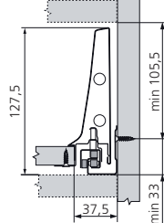
Maatvoeringen nodige inbouwruimte
