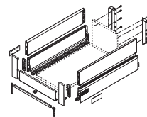
X = binnenbreedte - 132 mm
