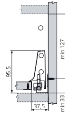
Nodige inbouwruimte
