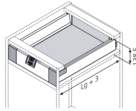
Inbouwruimte
