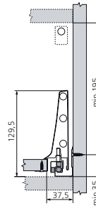
Nodige inbouwruimte
