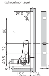
Boormaten front (schroefmontage)
