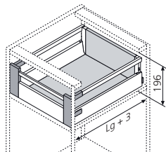
Inbouwruimte
