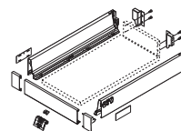
X = binnenbreedte - 132 mm
