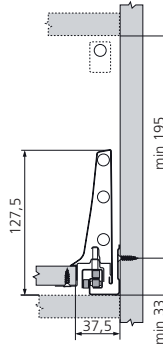
Maatvoeringen nodige inbouwruimte
