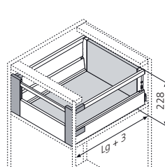
Inbouwruimte
