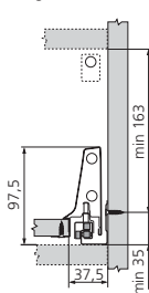
Nodige inbouwruimte
