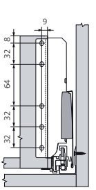
Inbouwmaten rugwand
