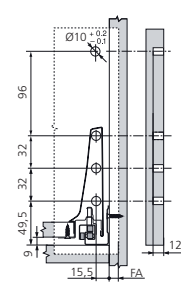
Inbouwmaten front (schroefmontage)
