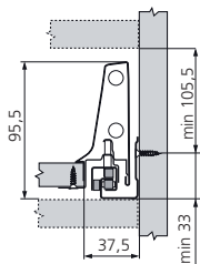
Maatvoeringen nodige inbouwruimte
