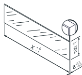
X = binnenbreedte - 118 mm
