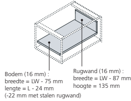
Maatvoeringen rugwand en bodem LW : corpusbinnenbreedte L : lengte lade
