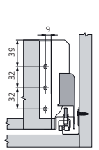
Inbouwmaten rugwand
