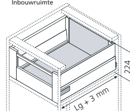
Inbouwruimte
