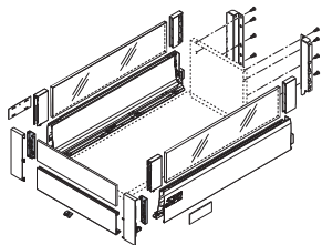
Inbouwruimte
