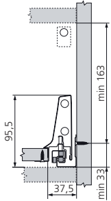
Maatvoeringen nodige inbouwruimte
