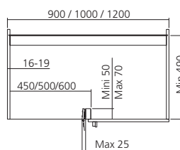
➔ Ensemble d'angle Slide Corner
