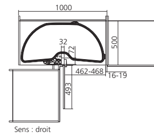
➔ Ensemble d'angle Power Slide
