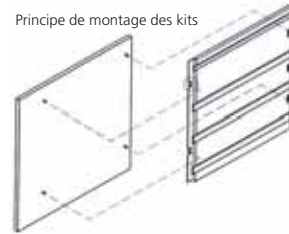
Fixation des kits
