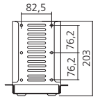
Montage sous plan de travail
