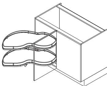
➔ Ensemble d'angle Twin Corner
