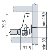
Côtes d'implantation du tiroir
