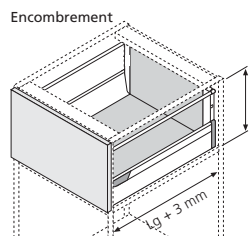
Lg : Longueur tiroir
