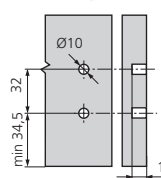
Côtes de perçage façade (pour montage INSERTA)
