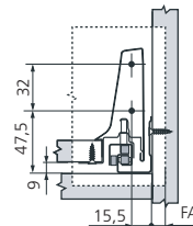
Côtes de montage façade (pour version à visser)
