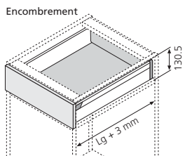
Encombrement
