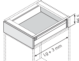
Encombrement
