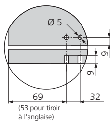
Perçage du fond
