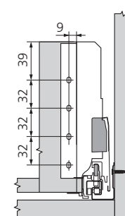
Côtes de montage dos
