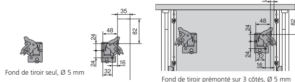
Encombrement
