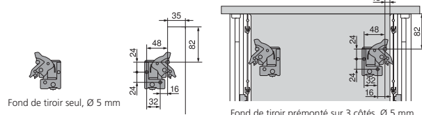
Fond de tiroir prémonté sur 3 côtés, Ø 5 mm
