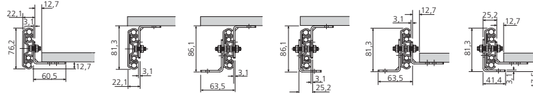
Montage avec la coulisse COU9301
