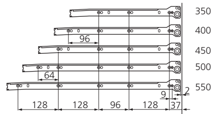
Fixation des coulisses corps de meuble
