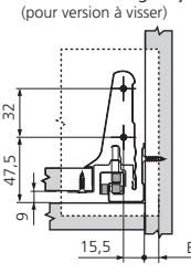
Côtes de montage façade (pour version à visser)
