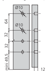
Côtes de perçage façade (pour montage INSERTA)
