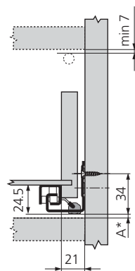
côtes du tiroir et montage de la coulisse
