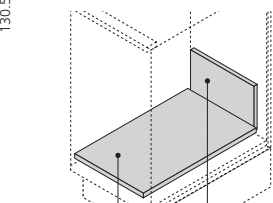
Fond (ep. 16 mm) : largeur = LW - 75 mm longueur = Lg - 24 mm Dos (ep. 16 mm) : largeur = LW - 87 mm hauteur = 116 mm
