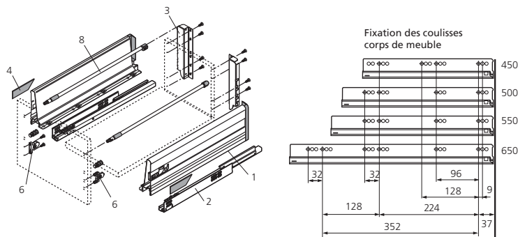
Encombrement
