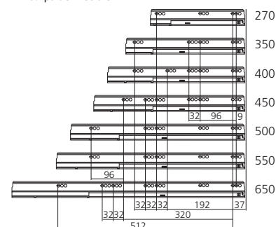
Fixation des coulisses corps de meuble
