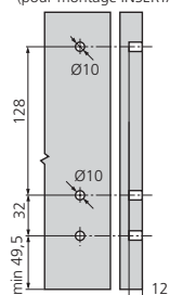
Côtes de perçage façade (pour montage INSERTA)
