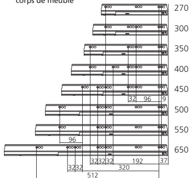
Fixation des coulisses corps de meuble
