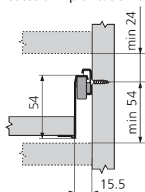
côtes d'implantation du tiroir
