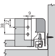
Côtes de montage dos
