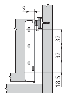
côtes de montage dos
