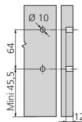
côtes de perçage façade (pour version à frapper, clipsable/expando)
