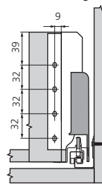
Côtes de montage dos
