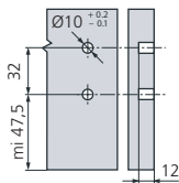
Côtes de perçage façade (pour montage INSERTA)
