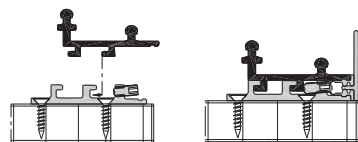
Montage des rails de roulement
