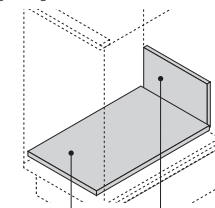
Fond (ep. 16 mm) : largeur = LW - 75 mm
