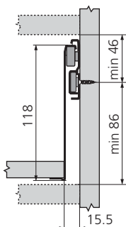
côtes d'implantation du tiroir
