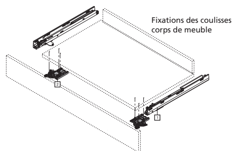
Position de montage de l'unité de verrouillage
