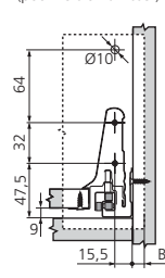
Côtes de montage façade (pour version à visser)
