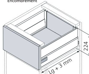
Encombrement
