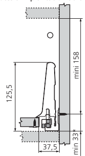
Côtes de perçage façade (pour montage INSERTA)
