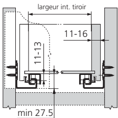
côtes du tiroir et montage de la coulisse
