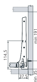
Côtes d'implantation du tiroir
