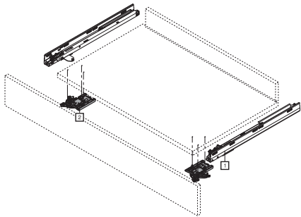
Position de montage de l'unité de verrouillage
