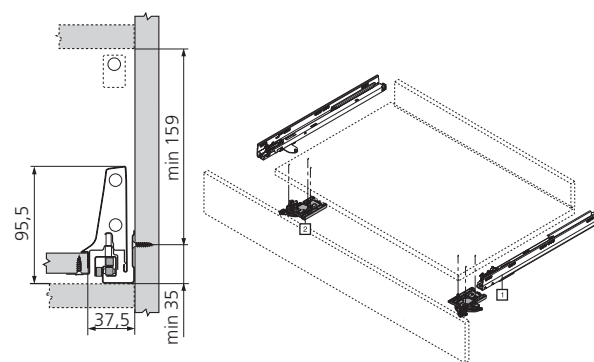
Position de montage de l'unité de verrouillage
