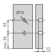
Côtes de perçage façade (pour montage INSERTA)
