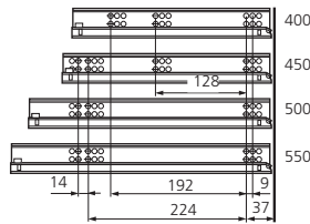
Côtes de débit fond et dos
