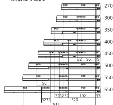
Fixations des coulisses corps de meuble
