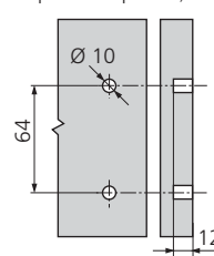
côtes de perçage façade (pour version à frapper, clipsable/expando)
