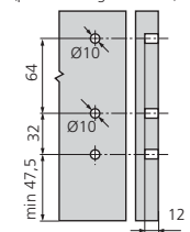
Côtes de perçage façade (pour montage INSERTA)
