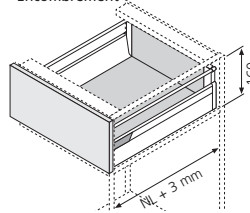
Lg : Longueur tiroir
