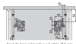
Fond de tiroir prémonté sur 3 côtés, Ø 5 mm
