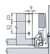
Côtes de montage dos
