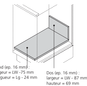
Côtes de débit fond et dos LW : largeur intérieure du corps de meuble Lg : Longueur tiroir
