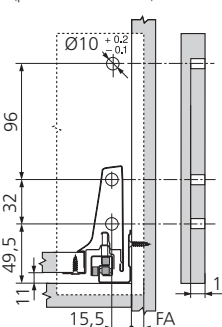
Côtes de montage façade (pour version à visser)
