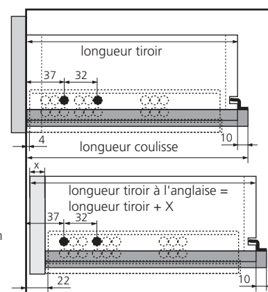
côtes du tiroir et montage de la coulisse
