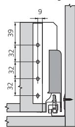
Côtes de montage dos
