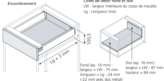
Côtes d'implantation du tiroir
