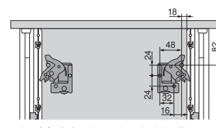
Fond de tiroir prémonté sur 3 côtés, Ø 5 mm Côtes de débit fond et dos LW : largeur intérieure du corps de meuble Lg : Longueur tiroir
