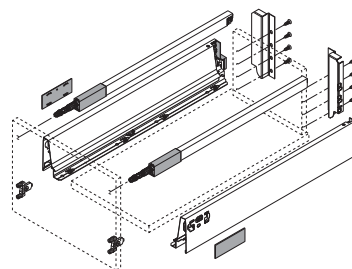
Fixation des coulisses corps de meuble
