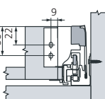
Côtes de montage dos
