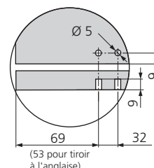
Perçage du fond
