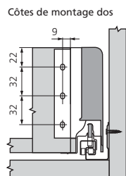
Côtes de montage dos
