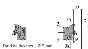
Fond de tiroir seul, Ø 5 mm
