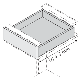
Encombrement
