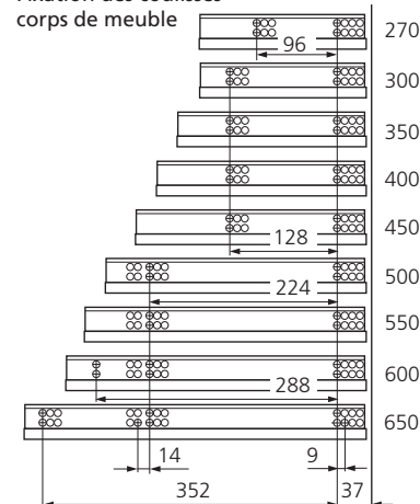
Fixation des coulisses corps de meuble
