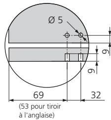
Perçage du fond
