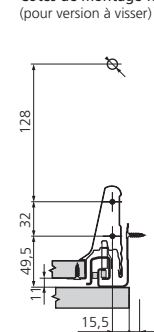
Côtes de montage dos
