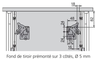
Fond de tiroir prémonté sur 3 côtés, Ø 5 mm
