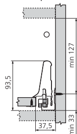
Côtes d'implantation du tiroir
