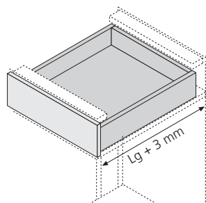
Encombrement
