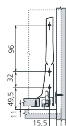
Côtes de montage façade (pour version à visser)
