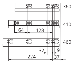
Fixation des coulisses corps de meuble
