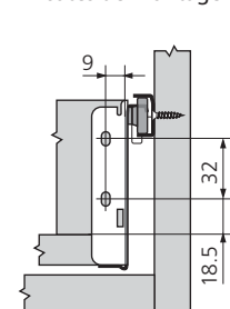
côtes de montage dos
