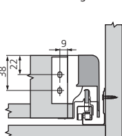
Côtes de montage dos
