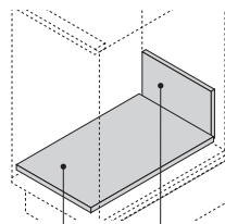
Fond (ep. 16 mm) : largeur = LW - 75 mm longueur = Lg - 24 mm (-22 mm avec dos métal) Dos (ep. 16 mm) : largeur = LW - 87 mm hauteur = 84 mm
