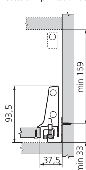
Côtes d'implantation du tiroir
