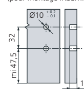
Côtes de perçage façade (pour montage INSERTA)
