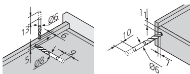
Usinage du tiroir bois
