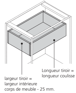
Fixation des coulisses corps de meuble
