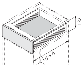
Encombrement
