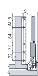
Côtes de montage dos
