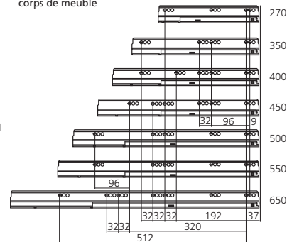
Côtes de débit fond et dos
