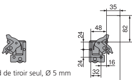
Fond de tiroir seul, Ø 5 mm
