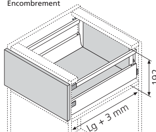
Encombrement
