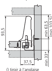
Côtes d'implantation du tiroir
