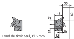
Fond de tiroir seul, Ø 5 mm
