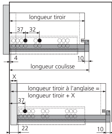
Encombrement
