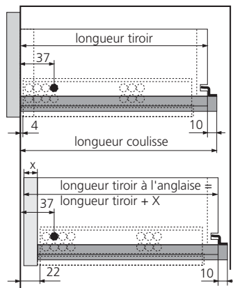
Encombrement
