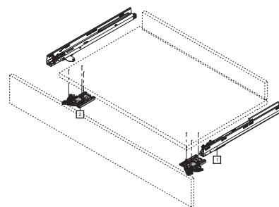
Position de montage de l'unité de verrouillage
