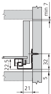
côtes d'implantation du tiroir
