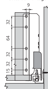
Côtes de montage dos
