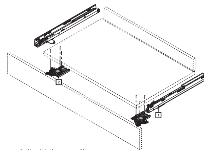
Position de montage de l'unité de verrouillage
