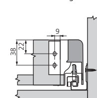
Côtes de montage dos
