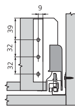
Côtes de montage dos
