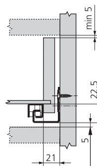
côtes d'implantation du tiroir
