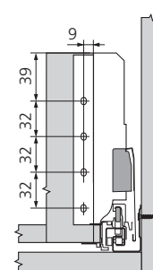
Côtes de montage dos
