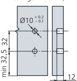
Côtes de perçage façade (pour montage INSERTA)
