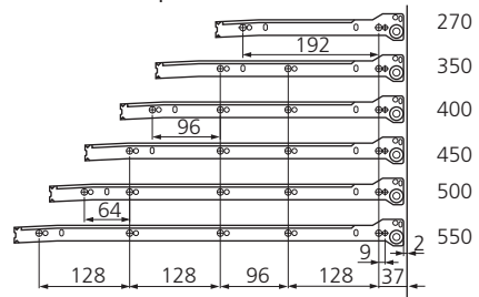
Fixation des coulisses corps de meuble
