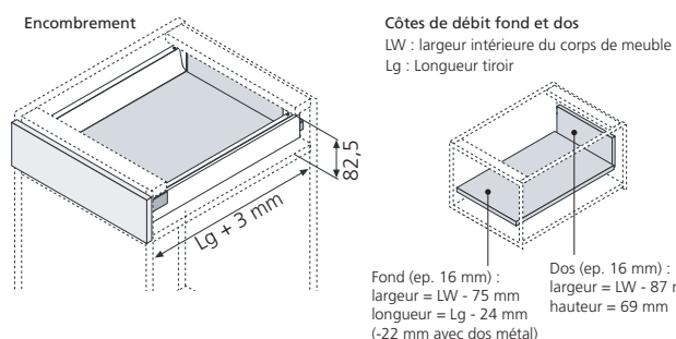
Côtes d'implantation du tiroir
