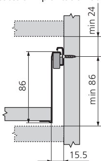
côtes d'implantation du tiroir
