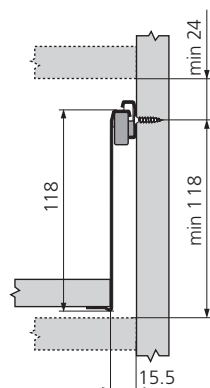
côtes d'implantation du tiroir
