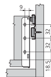
côtes de montage dos
