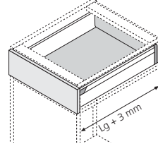
+ 40 mm pour tiroir à l'anglaise Lg : Longueur tiroir
