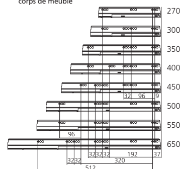
Fixation des coulisses corps de meuble
