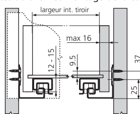
côtes du tiroir et montage de la coulisse
