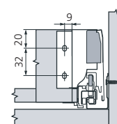
Côtes de montage dos
