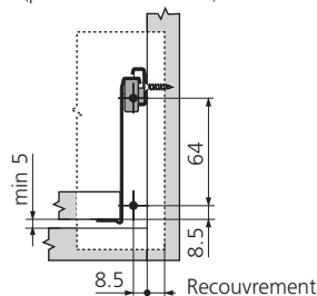
côtes de montage façade (pour version à visser)
