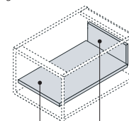
Côtes de débit fond et dos
