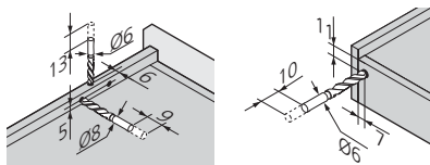
Usinage du tiroir bois
