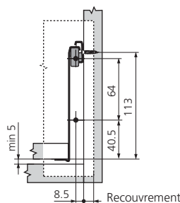
côtes de montage façade (pour version à visser)
