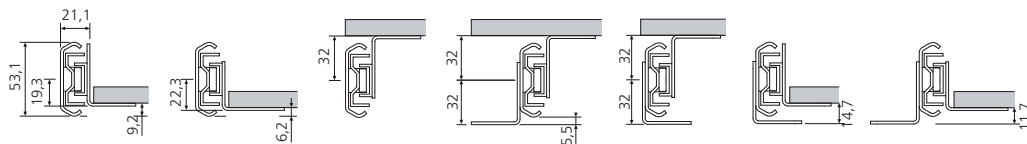
Montage avec la coulisse COU5321A
