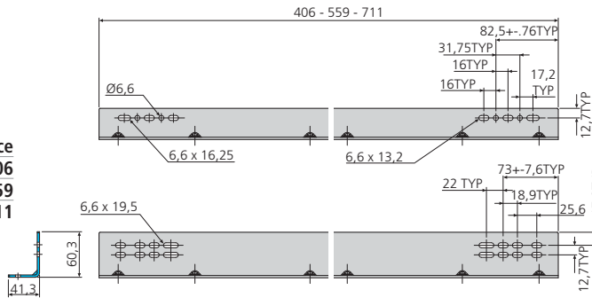
Montage avec la coulisse COU9301
