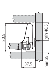
Côtes d'implantation du tiroir
