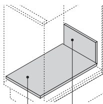
Fond (ep. 16 mm) : largeur = LW - 75 mm longueur = Lg - 24 mm Dos (ep. 16 mm) : largeur = LW - 87 mm hauteur = 167 mm
