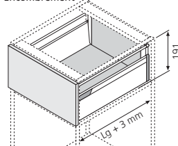
Lg : Longueur tiroir
