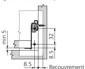
côtes de montage façade (pour version à visser)
