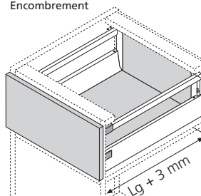
Encombrement
