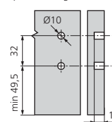
0) tiroir à l'anglaise
