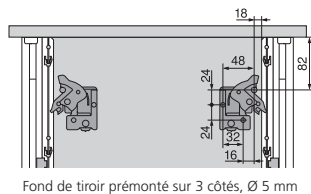
Fond de tiroir prémonté sur 3 côtés, Ø 5 mm
