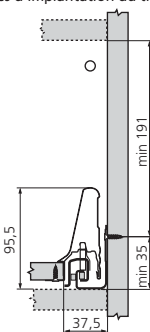
Côtes de perçage façade (pour montage INSERTA)
