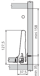
Côtes de perçage façade (pour montage INSERTA)
