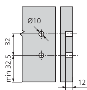
Côtes de perçage façade (pour montage INSERTA)
