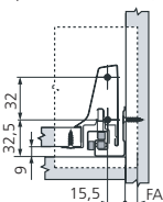
Côtes de montage façade (pour version à visser)
