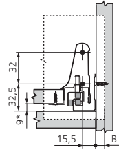
Côtes de montage façade (pour version à visser)
