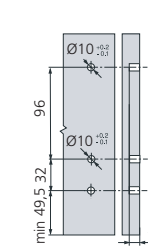
Côtes de perçage façade (pour montage EXPANDO)
