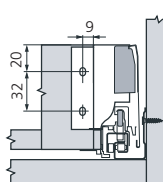
Côtes de montage dos
