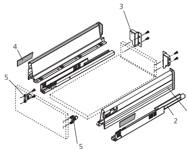
Fixation des coulisses corps de meuble
