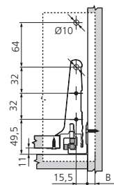
Côtes de montage dos
