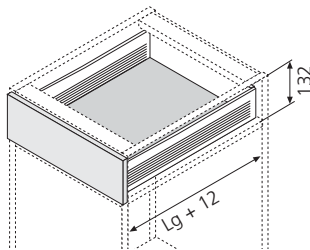
Encombrement
