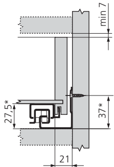
côtes d'implantation du tiroir
