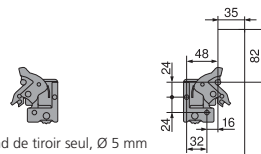
Fond de tiroir seul, Ø 5 mm
