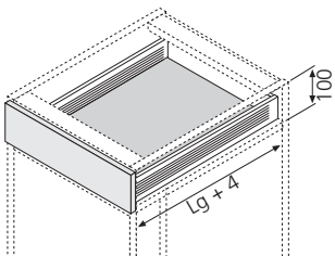
Encombrement
