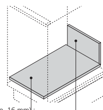
Fond (ep. 16 mm) : largeur = LW - 75 mm longueur = Lg - 24 mm (-22 mm avec dos métal) Dos (ep. 16 mm) : largeur = LW - 87 mm hauteur = 135 mm
